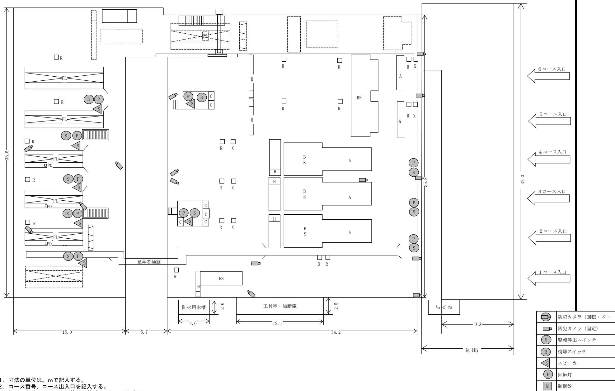
審査上屋及び審査機器配置図-1
