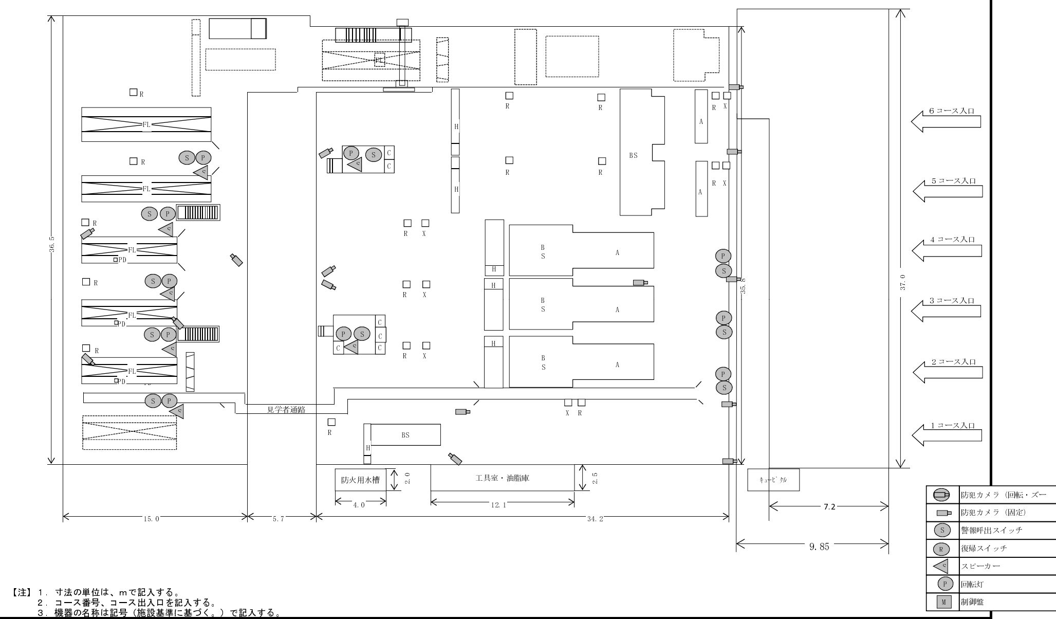
審査上屋及び審査機器配置図-1
