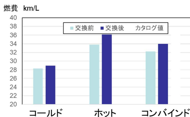
JC08 モード試験での比較
