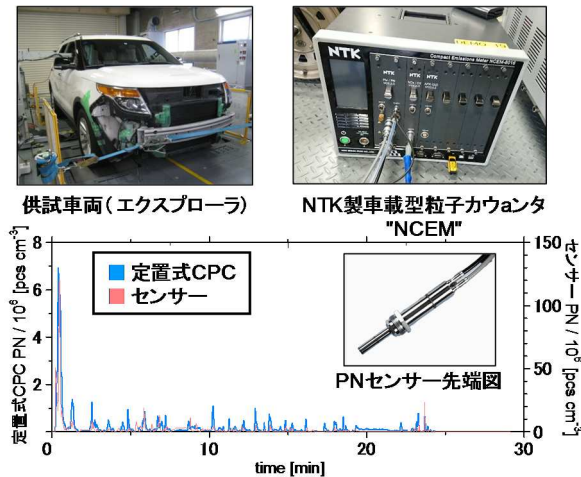
WLTC モード走行時における PN 排出挙動
