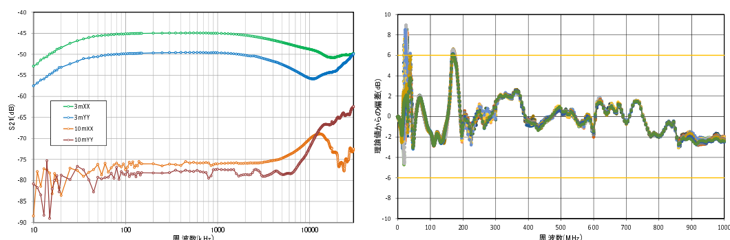
実車暗室の 30MHz 以下の磁界特性測定例 ESA 暗室の性能評価測定例
