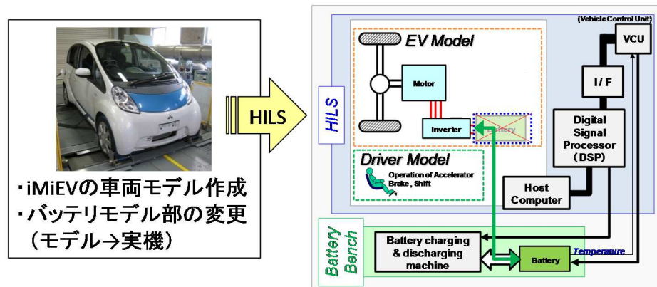
バッテリーHILS の構築
