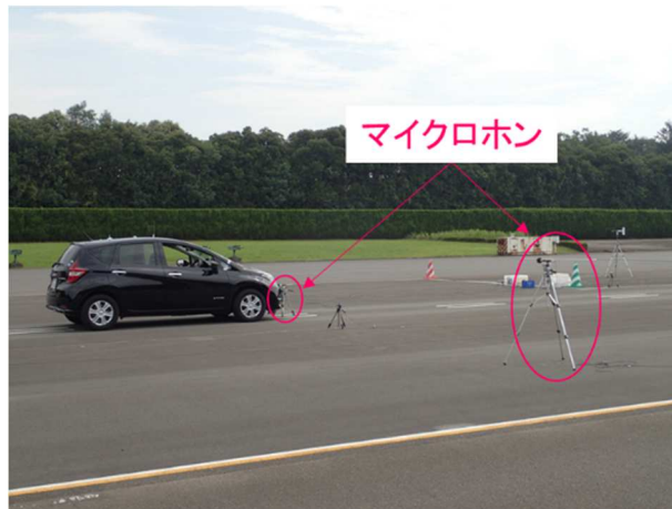
音モデルの一つであるパワートレイン系騒音の測定の様子
