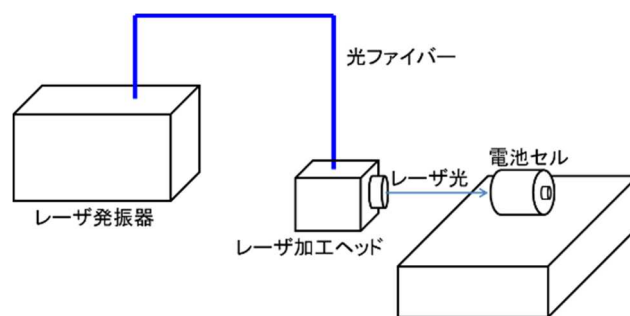
レーザーイニシエーションの模式
