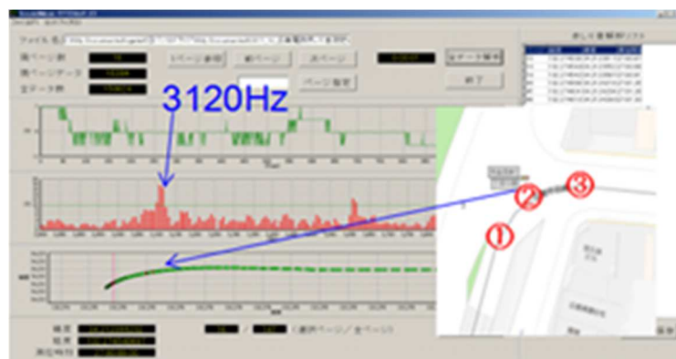
走行音データの分析によるきしり音発生箇所の特定
