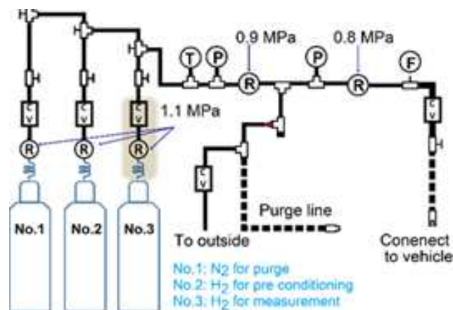
水素供給配管の模式
