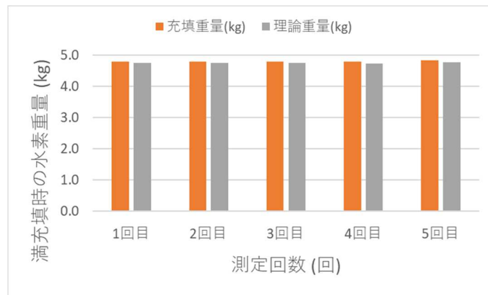
水素充填重量（実測値）と圧力から求めた理論重量との比較
