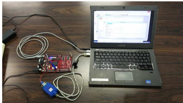
ハッシュ関数を使用した ECU ソフトウェアの検査実験装置
