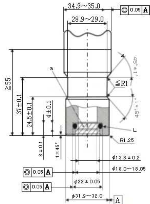
図 2: M2、M3、N2 および N3 車両の 20 MPa 充填装置サイズ 2 (レセプタクル) Figure 2: 20 MPa Filling unit Size 2 (receptacle) for M2, M3, N2 and N3 vehicles
