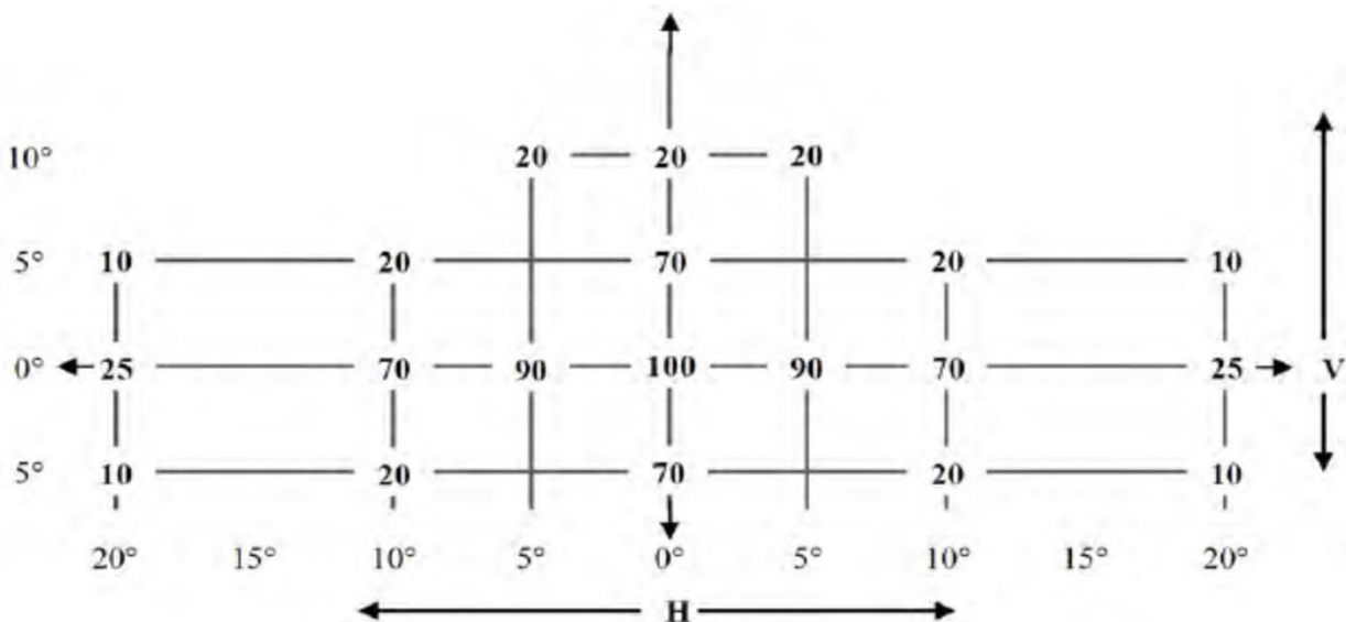
図 A3-II：デイトイムランニングランプの配光
