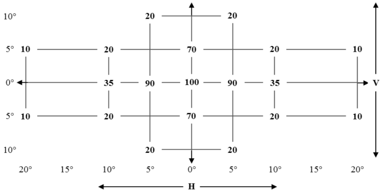
図A3-I フロントおよびリアポジションランプ、パーキングランプ、 エンドアウトラインマーカールンプ、ストップランプおよび方向指示器の標準配光 Figure A3-I Standard light distribution for front and rear position-, parking-, end-outline marker-, stop- and direction indicator lamps
