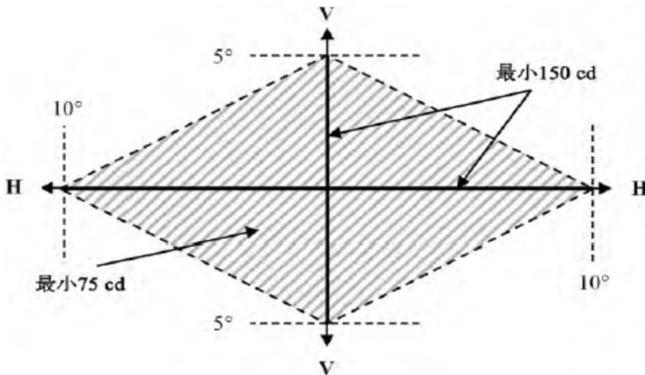
図 A3-VI : リアフォグランプの配光
