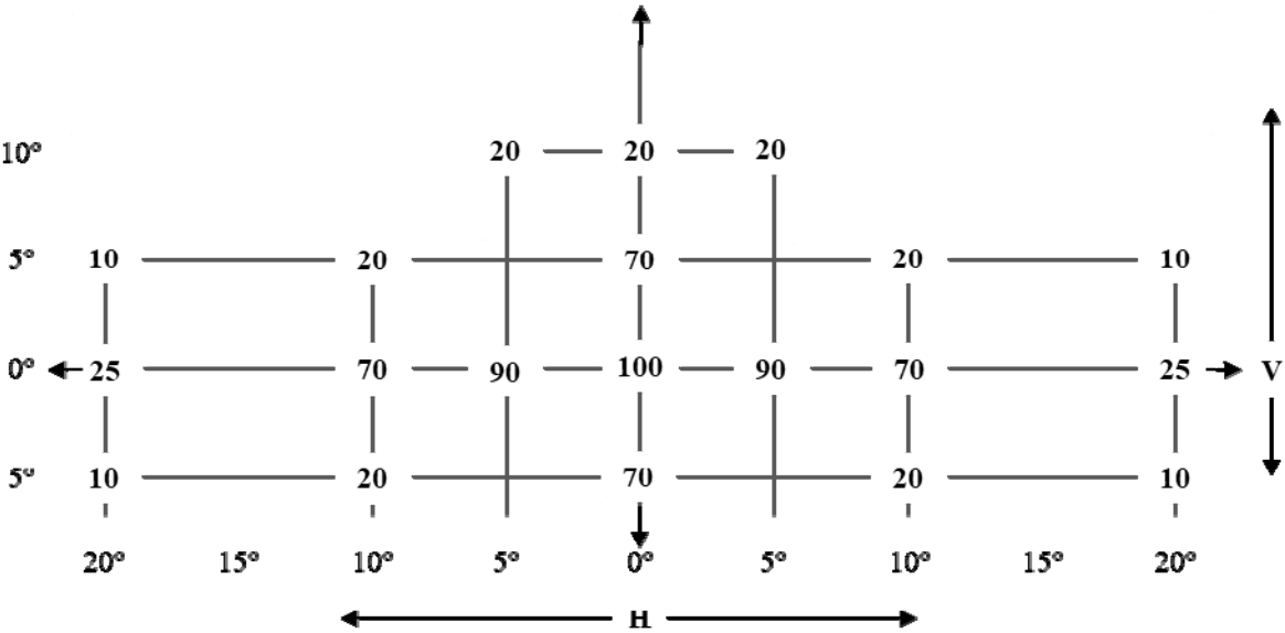
図A3-II デイタイムランニングランプの配光 Figure A3-II Light distribution for daytime running lamps
