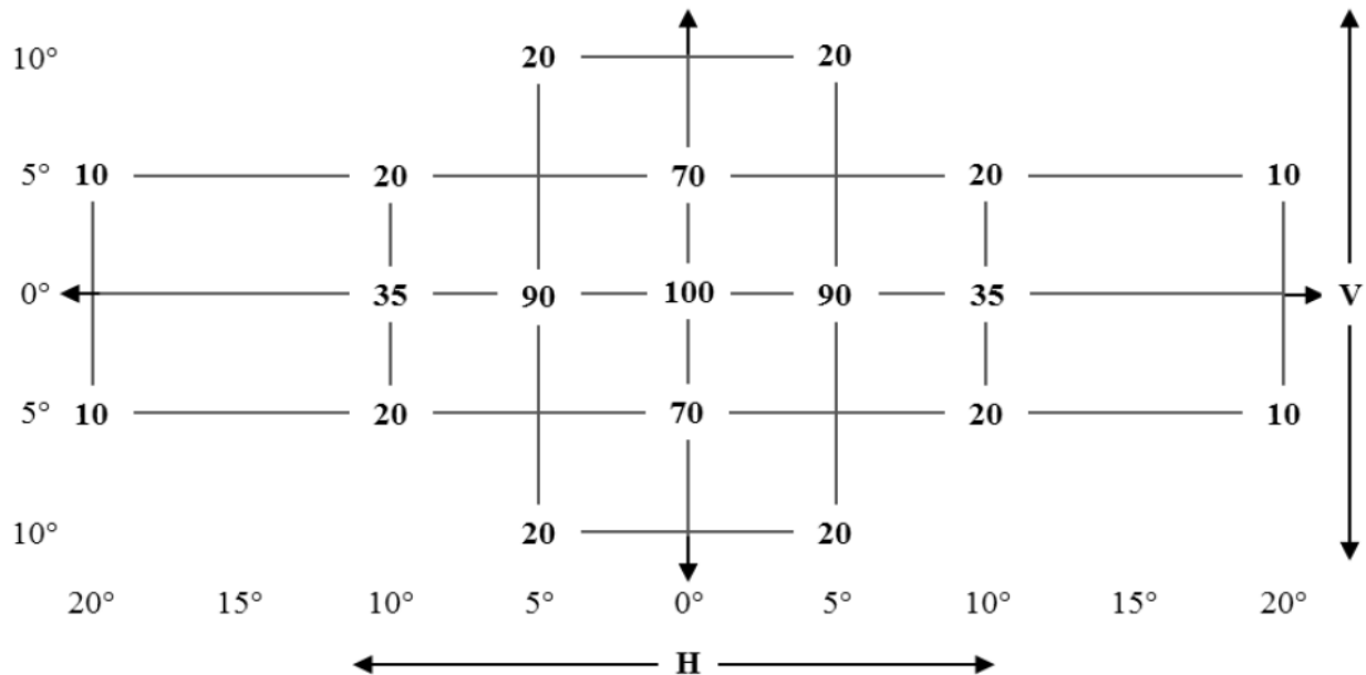
図A3-I フロントおよびリアポジションランプ、パーキングランプ、 エンドアウトラインマーカールランプ、ストップランプおよび方向指示器の標準配光 Figure A3-I Standard light distribution for front and rear position-, parking-, end-outline marker-, stop- and direction indicator lamps
