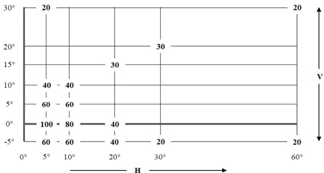
図A3-IV: カテゴリー6方向指示器の配光 Figure A3-IV: Light distribution for direction indicator lamps category 6
